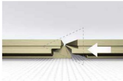
Горизонтальное соединение
